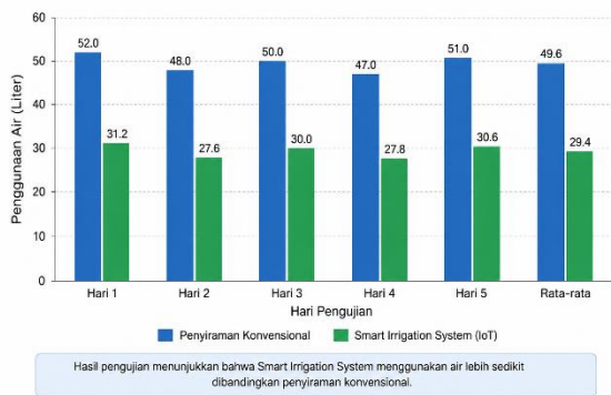
Gambar 9. Perbandingan Penggunaan Air
