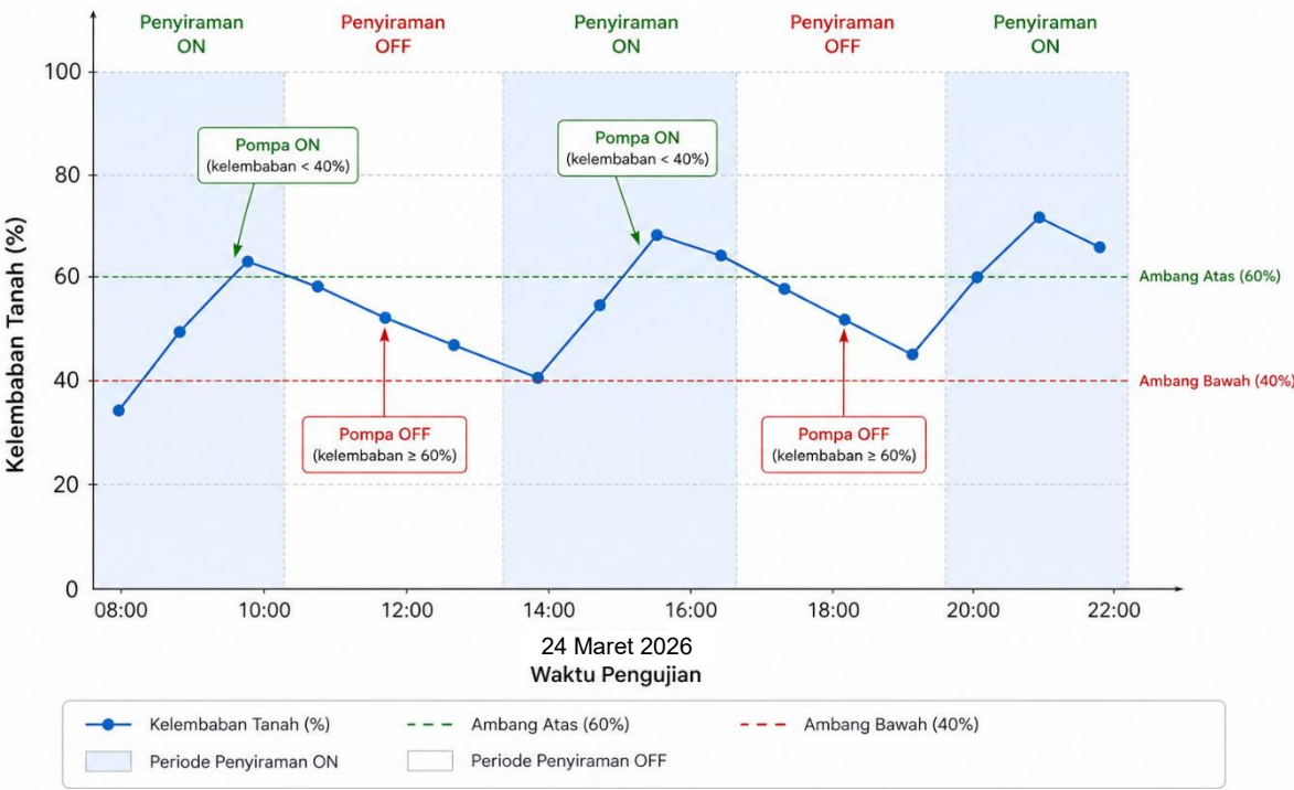
Gambar 7. Grafik Kelembaban Tanah
