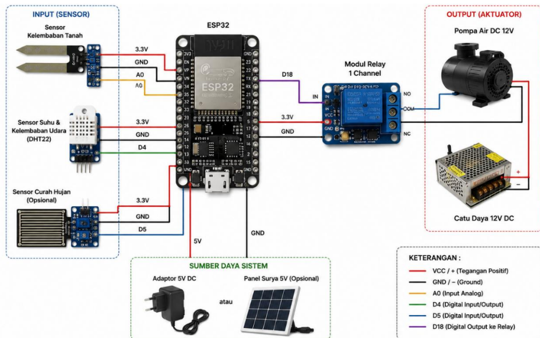
Gambar 5. Rangkaian Hardware Sistem
