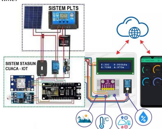
Gambar 1. Skema sistem stasiun cuaca berbasis IoT
